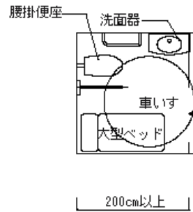
○ 大型ベッド付便房
