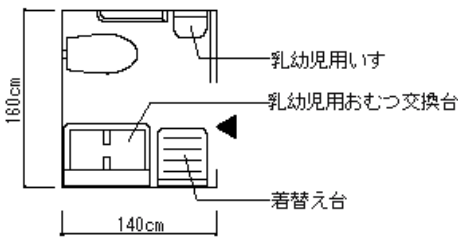
○ 乳幼児連れに配慮した便房の寸法 (ベビーカーと共に入ることができる寸法)
