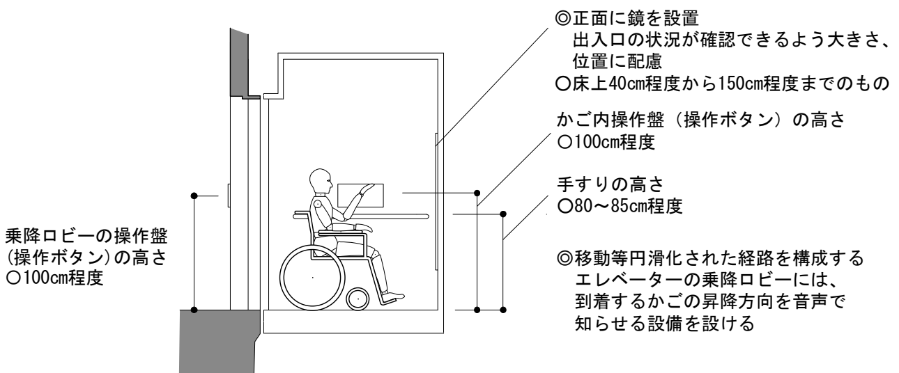
参考 2-1-24 : エレベーターの断面の例
