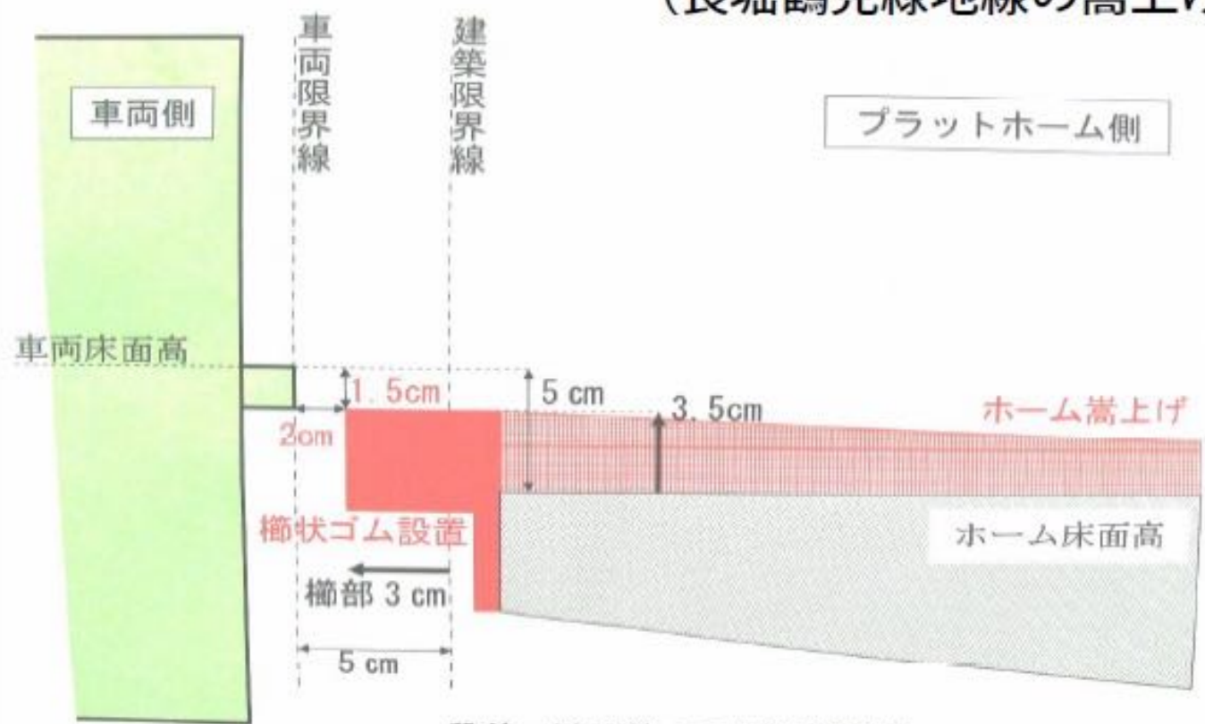
段差・隙間縮小の標準断面図
