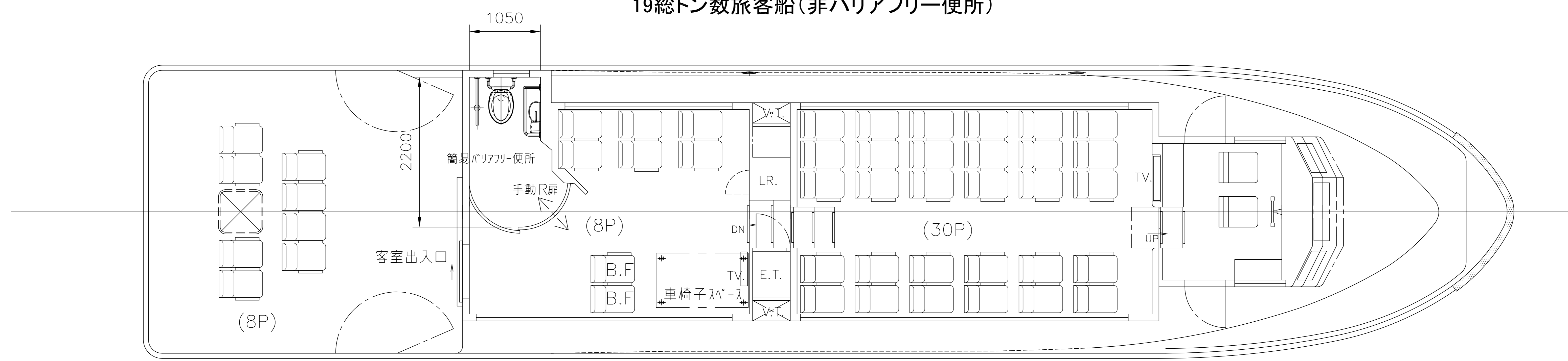
19総トン数旅客船試設計(B型オプション2手動R扉)
