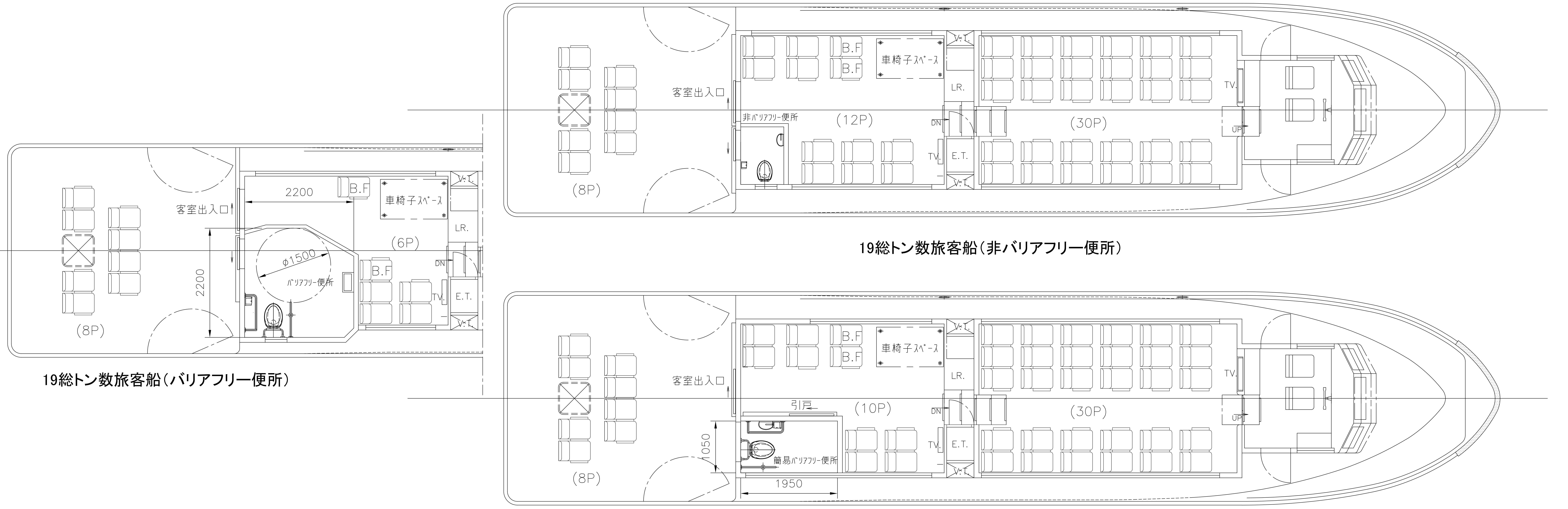
19総トン数旅客船試設計(簡易バリアフリー便所B型引戸)
