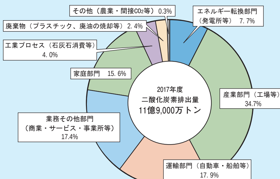
日本の二酸化炭素排出量（部門別）2017年度
