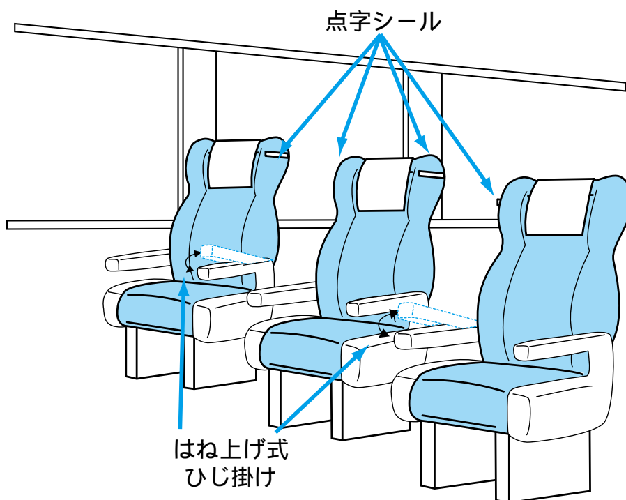
3列シートの場合
