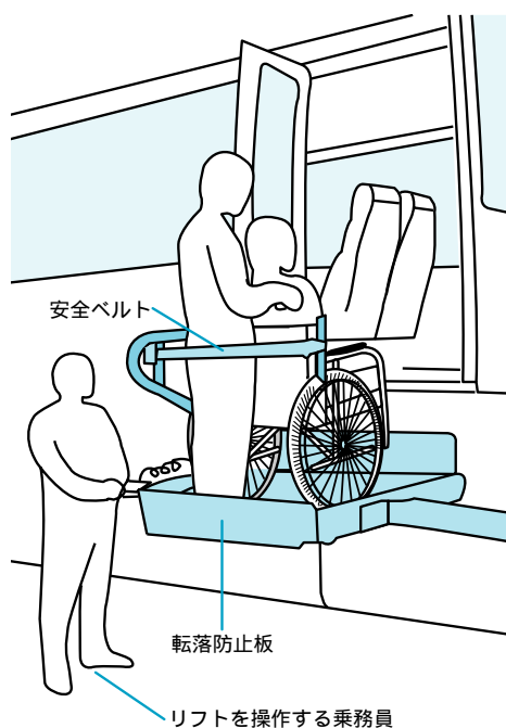
乗降用リフトの使用例(1)
