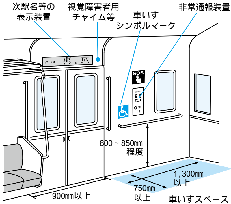
車いすスペースの設置例
