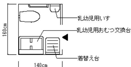
○乳幼児連れに配慮した便房の寸法 (ベビーカーと共に入ることができる寸法)
