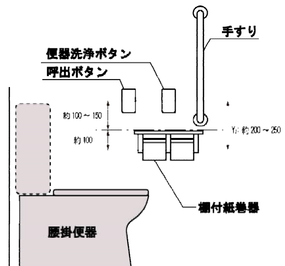
②棚付紙巻器を設置する場合
