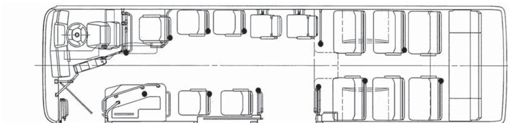
参考 4-2-2：中型ノンステップバスの平面図
