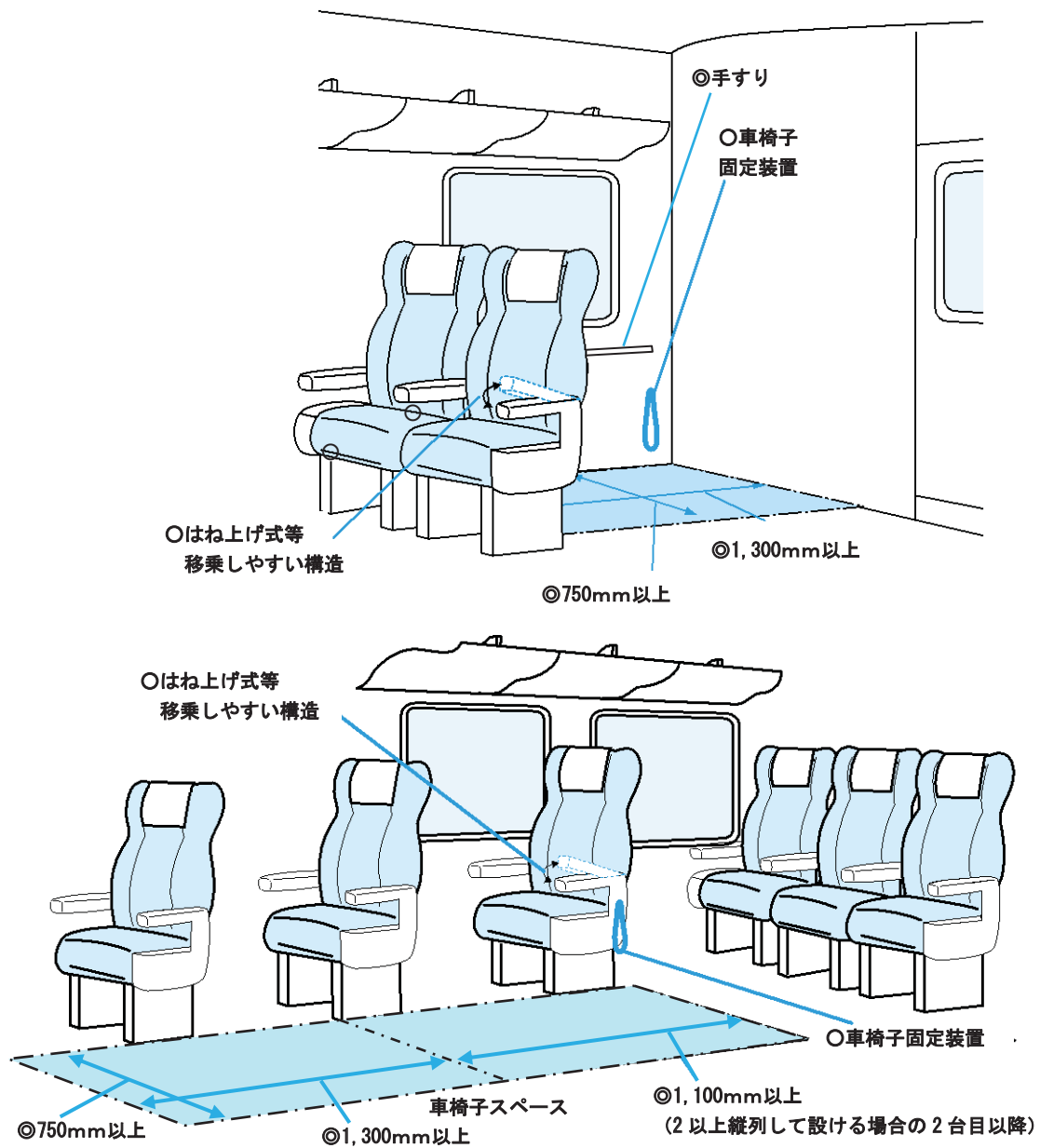
参考 4-1-42：車椅子スペースの例（新幹線車両を除く）
